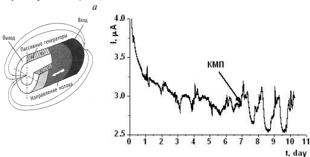
Рис.1. Концентратор магнитного поля, патент RU 2154870 С1, 20.08.2000 Бюл.№23 – а; изменение характера вариации тока в ЭХ ячейке с водой в присутствии КМП – б
