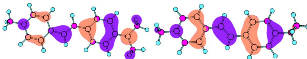
Рис. 1. Расчётные структуры ВЗМО катионной части DAST и его протонированной формы.
