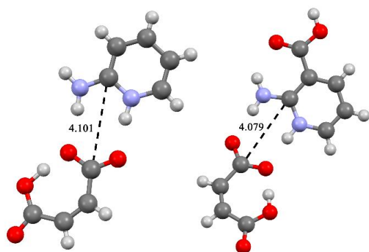
Рис.1 Структура гетеродимеров [2AmPyr + Mle] и [2AmNic + Mle]. Прерывистая линия обозначает расстояние между атомами углерода групп H 2 N-C-NH и CO 2 - , R(H 2 N-C-NH...CO 2 - ).
