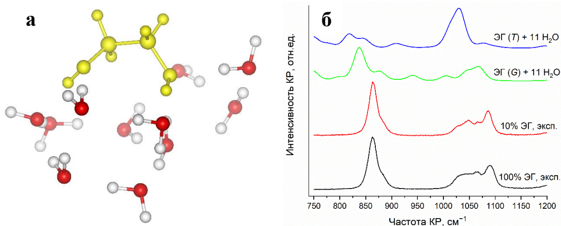
Рис. 1. Данные квантово-химического моделирования для водных растворов ЭГ: а — структура кластера, содержащего молекулу ЭГ в gauche -конформации (выделена жёлтым цветом) и 11 молекул воды; б — теоретические спектры КР систем ЭГ-вода, содержащих 1 молекулу ЭГ в gauche - или trans -конформации, а также 11 молекул воды, приведённые в сравнении с экспериментальными спектрами КР чистого жидкого ЭГ и 10%-ного водного раствора ЭГ
