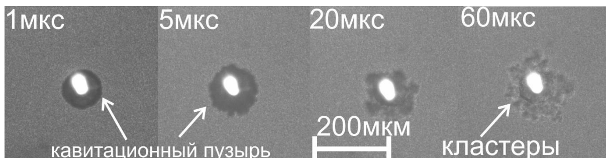
Рис.1. Эволюция кавитационных пузырей в жидком диоксиде углерода (80 бар, 300К) после воздействия наносекундного (6 нс, 400 мкДж) лазерного импульса. Задержки между силовым и пробным импульсом указаны на рисунке
