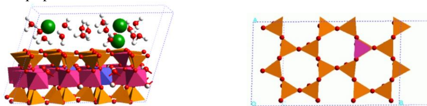
Рис.1. Модель кристалла набухающей глины (монтмориллонита) с ионами \text{Na}^+ и молекулами \text{H}_2\text{O} на поверхности. Справа показан вид сверху на силиоксановую поверхность кристалла. Изоморфные замещения в каждом слое выделены другим цветом.
