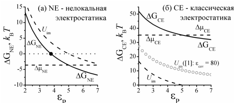
Рис. Зависимость изменения свободной энергии \Delta G_{NE} и \Delta G_{CE} (формулы (5), сплошные кривые) перехода катиона K + из свободного раствора в центр сферической водной полости радиуса 5Å от диэлектрической проницаемости \epsilon_p окружающей полость среды.
