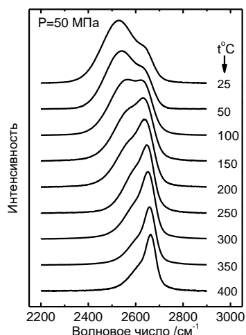
Рис.1. Спектры комбинационного рассеяния раствора \text{NaClO}_4 в \text{H}_2\text{O}
