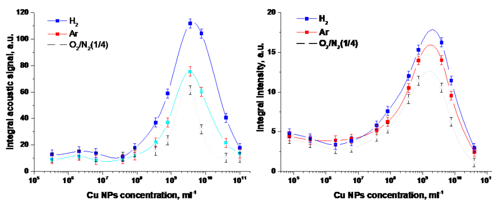
Рис.1 Влияние растворенных в воде газов на интенсивность (А) интегральных акустических сигналов и (В) светимости плазмы в зависимости от концентрации наночастиц Cu.
