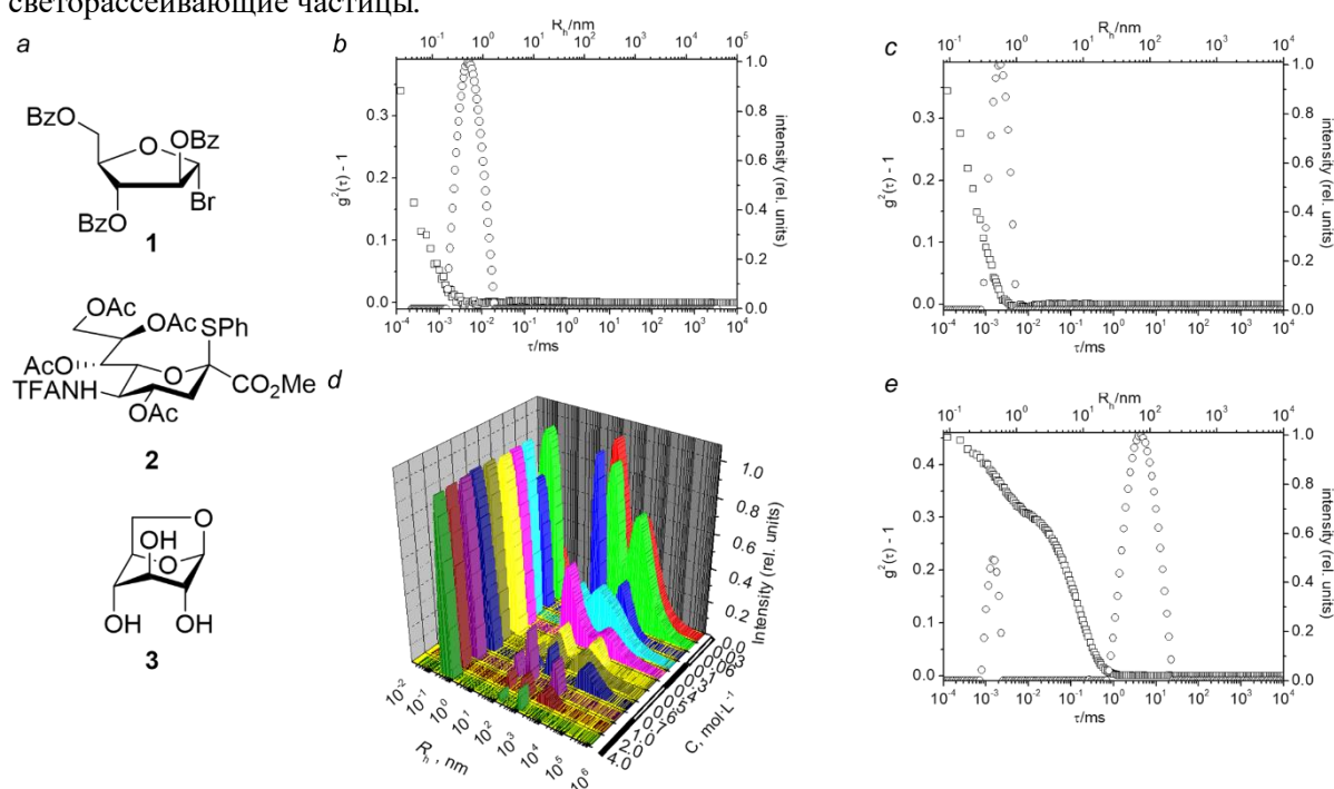
Рис. 1. Структуры исследуемых соединений (a). Корреляционные функция и распределения по размерам для 100 мМ растворов 1 в MeCN (c) и 1,2 дихлорэтане (e) [5], для 86 м М раствора 2 в MeCN (b) [4]. Зависимость распределения по размерам для водных растворов 3 от концентрации (0.03–4 М) (d) [3].
