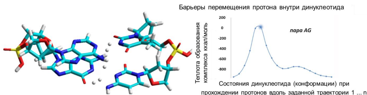
Рис. 1 Продольные водородные связи в ДНК (результаты квантовохимического моделирования динуклеотида).
