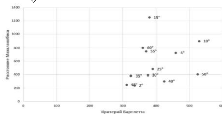
Рис.1. Диаграмма рассеяния с центрами состояний воды при различных температурах.
